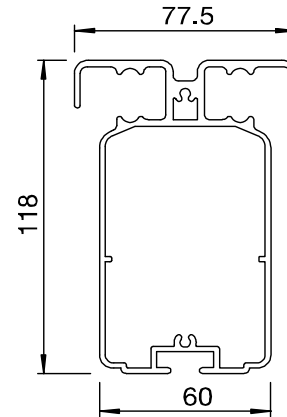
Führungsschiene PS-699
