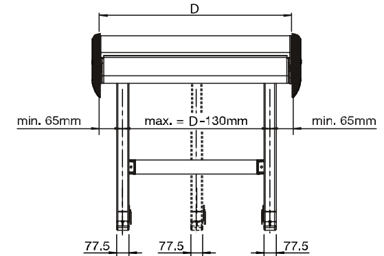
Querstrebe
