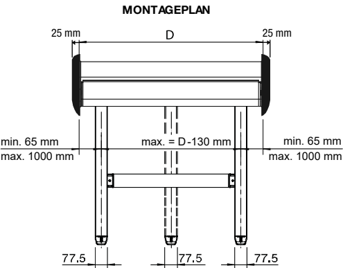
D plus Abdeckkappe 25 mm je Seite
