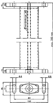
B-Winkel PS-547 -Höhe auf Maß- max. 350 mm
