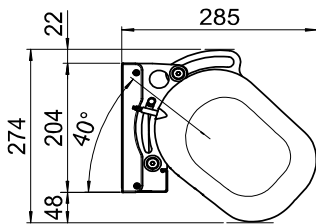
MIT 40° NEIGUNG
