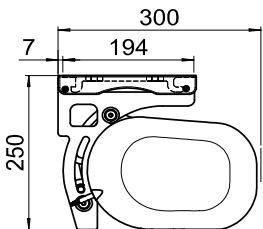
DECKENMONTAGE
