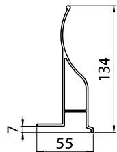
B-403 TUCHWELLENBLLENDE
