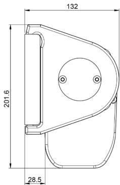
Wandmontage mit Motor 90°
