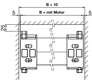
Montage in Nische (mit Motor)
