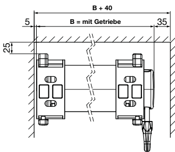
Montage in Nische (mit Getriebe)
