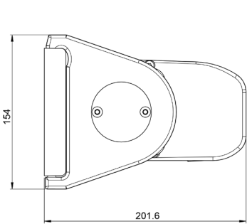
Wandmontage mit Motor 3°
