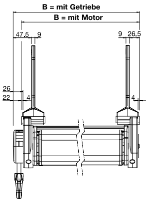
Montageplan
