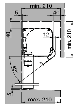
MONTAGEPLAN (LAIBUNGSMONTAGE) VIA DIREKTVERSCHRAUBUNG
