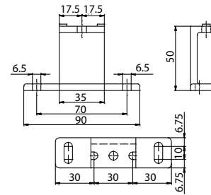
B-Winkel FS-602-1 für 1 Führung
