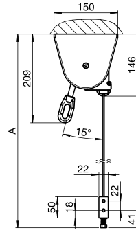
Deckenmontage
