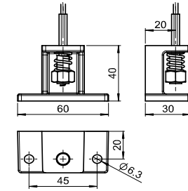
B-Winkel für Bodenbefestigung US-120-1
