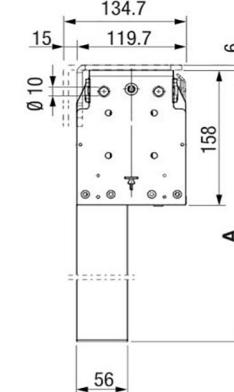
Zweiteilige Führung
