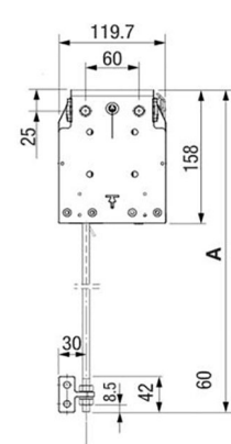
Stangenführung VA214-2
