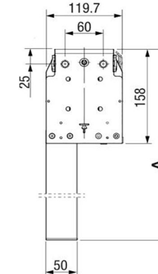
Einteilige Führung
