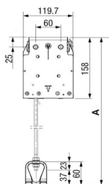
Stangenführung VA201-2
