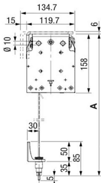
Seilführung VA212-1
