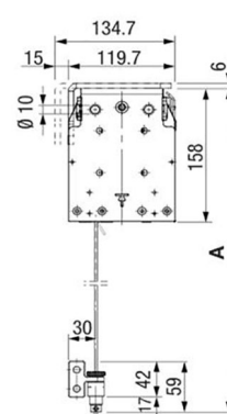
Seilführung VA214-1
