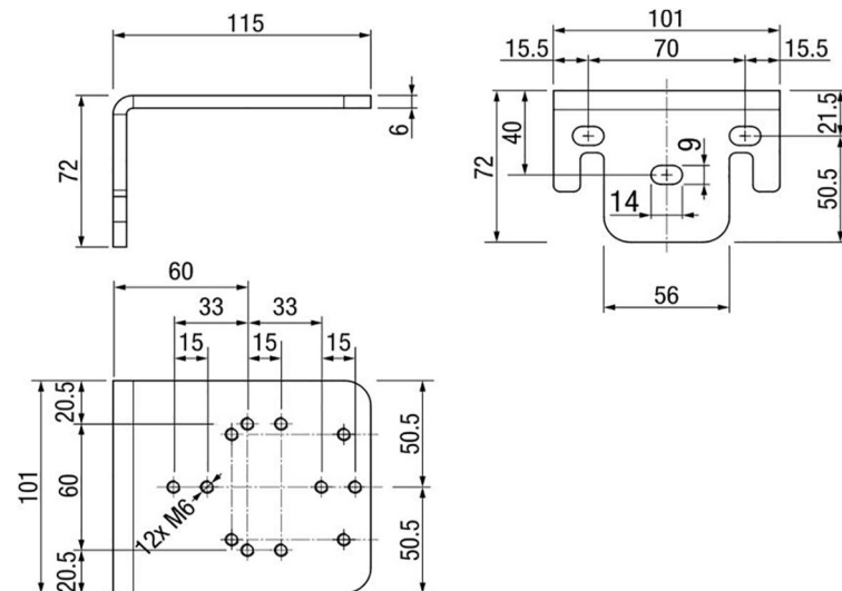
VA301 Wandkonsole
