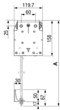
Stangenführung VA212-2
