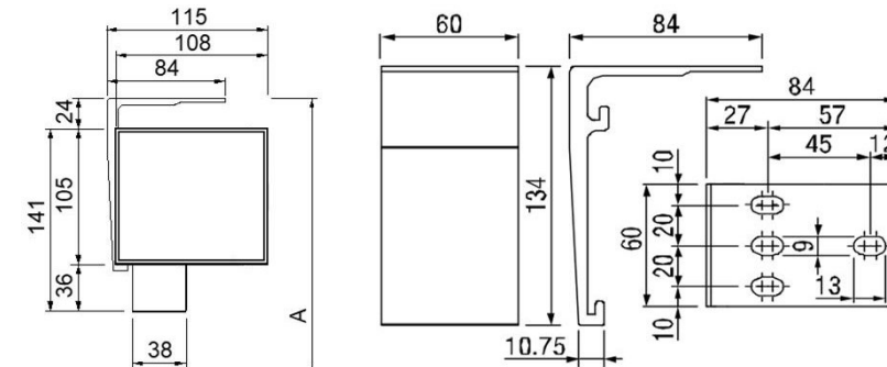
VA211-1 Deckenkonsole hoch
