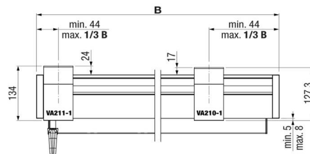
Verschieberegion Deckenkonsol VA210-1 / VA211-1
