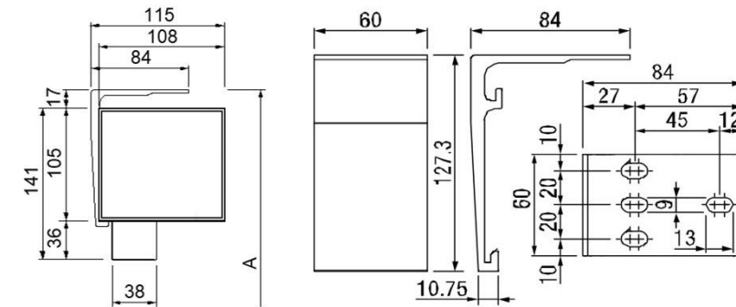
VA210-1 Deckenkonsole flach*
