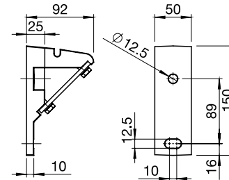
S-831-5 Wand-/Deckenkonsole spezial (schmal von vorne) Nicht möglich bei SELECT-PLUS / SELECT mit AV!
