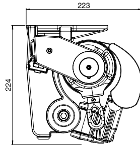
S-8130 Deckenmontage
