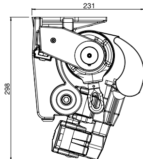
Deckenmontage
