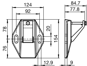
S-821-1 Wand-/Deckenkonsole
