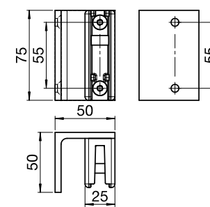
SR-418 Befestigungswinkelsatz
