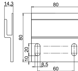
SR-606 Wandkonsole
