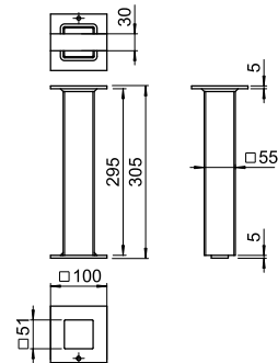
SR-413-2 Bodenhülse
