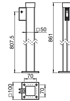
SR-415-1 Aufschraubpfosten
