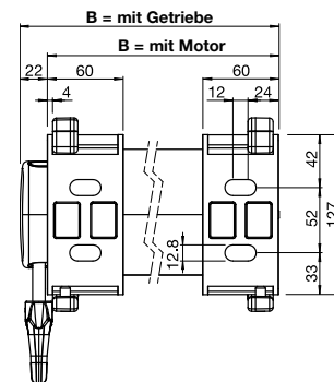
Montageplan
