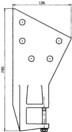
Dachsparren-Konsole S-225
