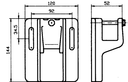
Wand-Decke S-221-1 Universalkonsole
