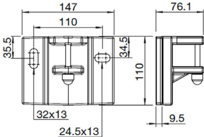
Wand-Spezial S-221-3-1
