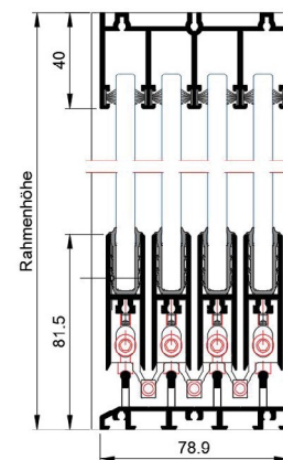
Abdeck-/Rahmenprofil 4-läufig.
