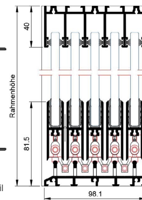
Abdeck-/Rahmenprofil 5-läufig.
