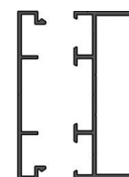
Abdeck-/Rahmenprofil 4-läufig.
