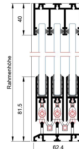
Abdeck-/Rahmenprofil 3-läufig.
