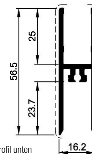
Flügelprofil unten
