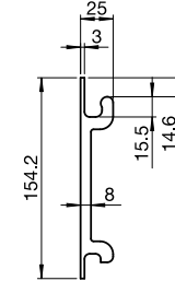
S-721-3 Profilkonsole
