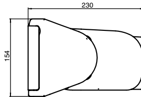
Wandmontage mit Motor 3° eckig
