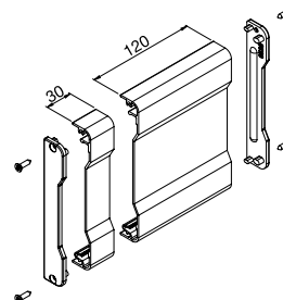
S-731-2 Konsolenabdeckung für Profilkonsole S-721-5
