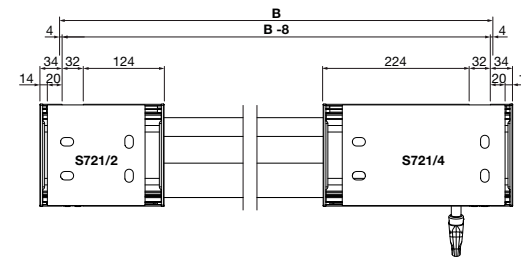
Montageplan (mit Konsolenabdeckung)
