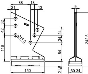
S-725 Dachsparrenkonsole
