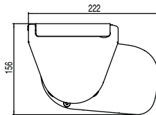
Deckenmontage mit Motor 5°
