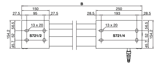
Montageplan (ohne Konsolenabdeckung)
