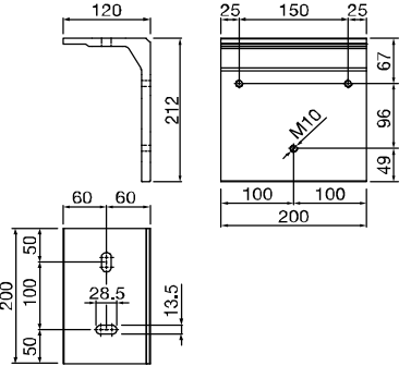
DACHSPARRENWINKEL BX-427
