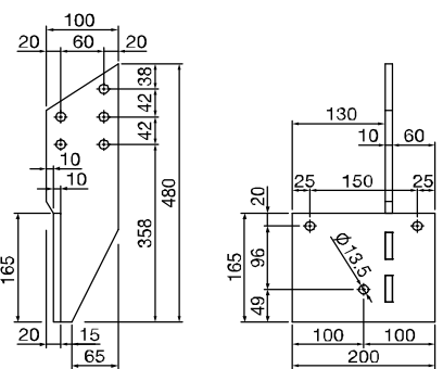
DACHSPARRENWINKEL BX-427
