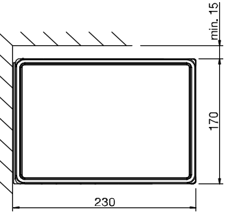
DECKENMONTAGE
