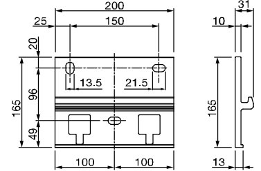
DECKENWINKEL BX-426
