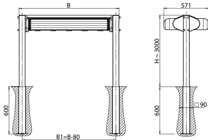
Mit Bodenhülse
