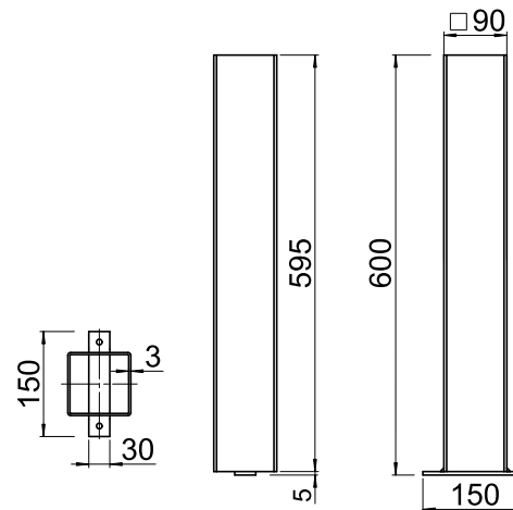
Bodenhülse
