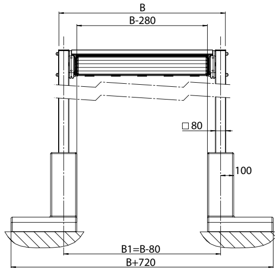
Mit Betonsockel
