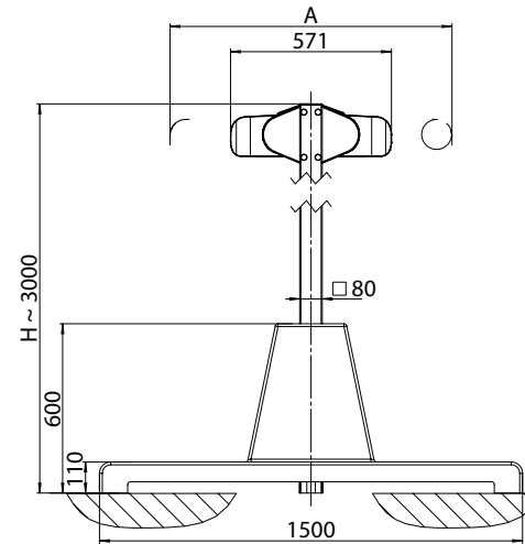
Mit Betonsockel
