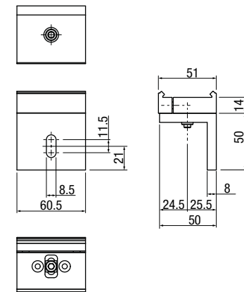
Befestigungshalter (Laibungsmontage)
