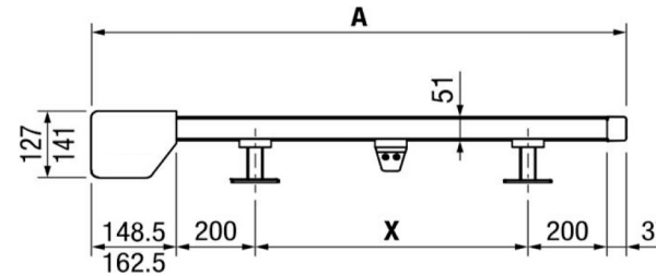
Seitenansicht (Freistehend)
