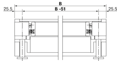
Frontansicht (Freistehend)
