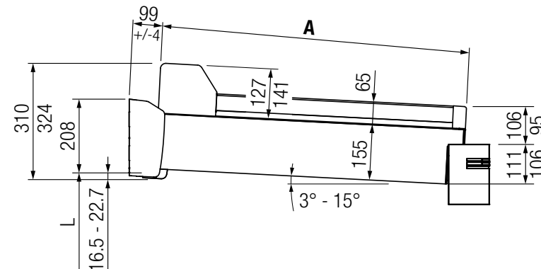
Seitenansicht (Montage auf NYON PLUS GP4100 / GP4200)
