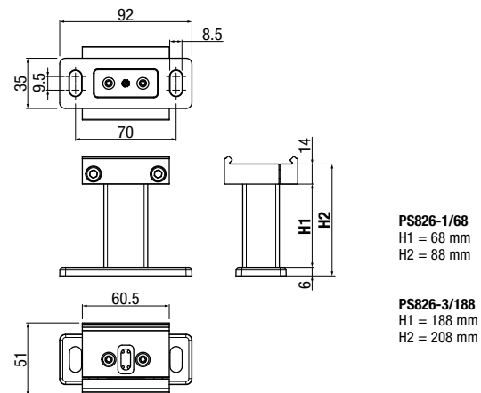
Befestigungshalter (Einfachplatte)
