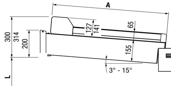
Seitenansicht (Montage auf NYON PLUS GP4100 / GP4200)
