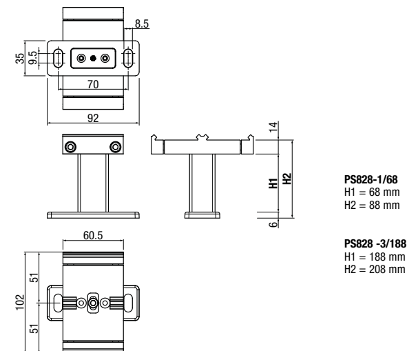
Befestigungshalter (Doppelplatte)
