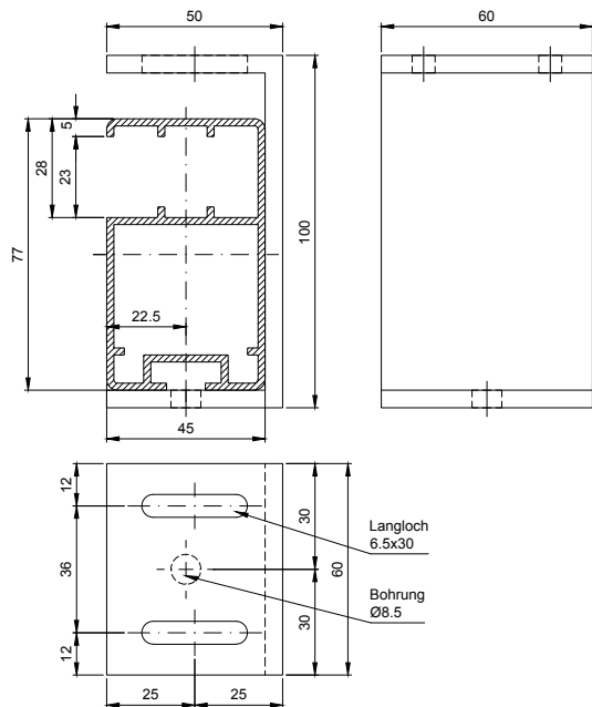
Seitenansicht
