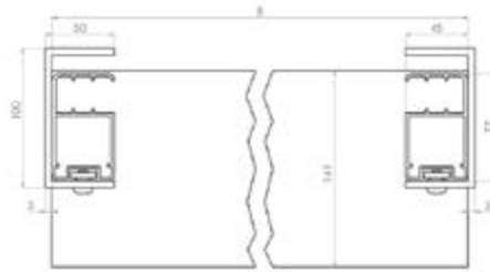
B: Totalbreite=Achsabstand Wintergartensprossen + 45 mm
